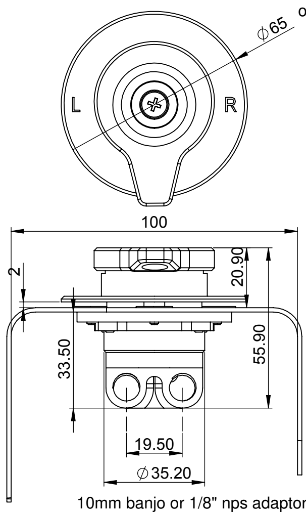
V6 - M10 PORTS MASS 127g
